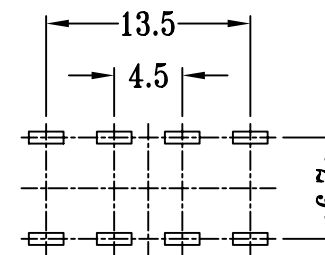
P.C.B LAYOUT
